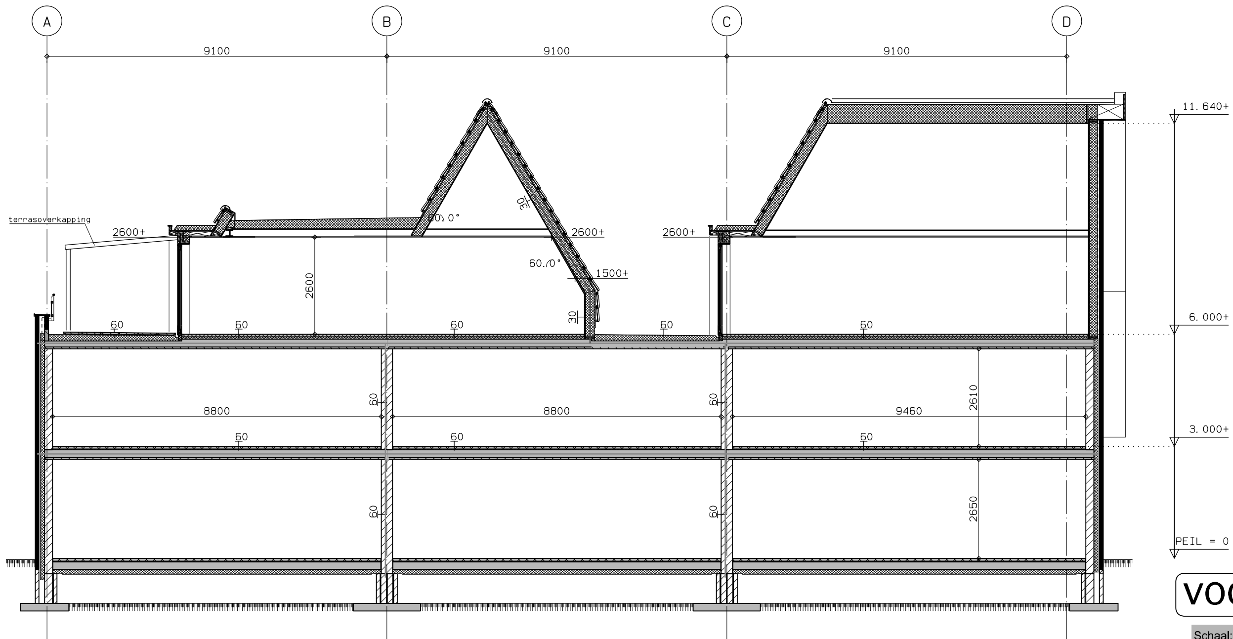
doorsnede A-A
