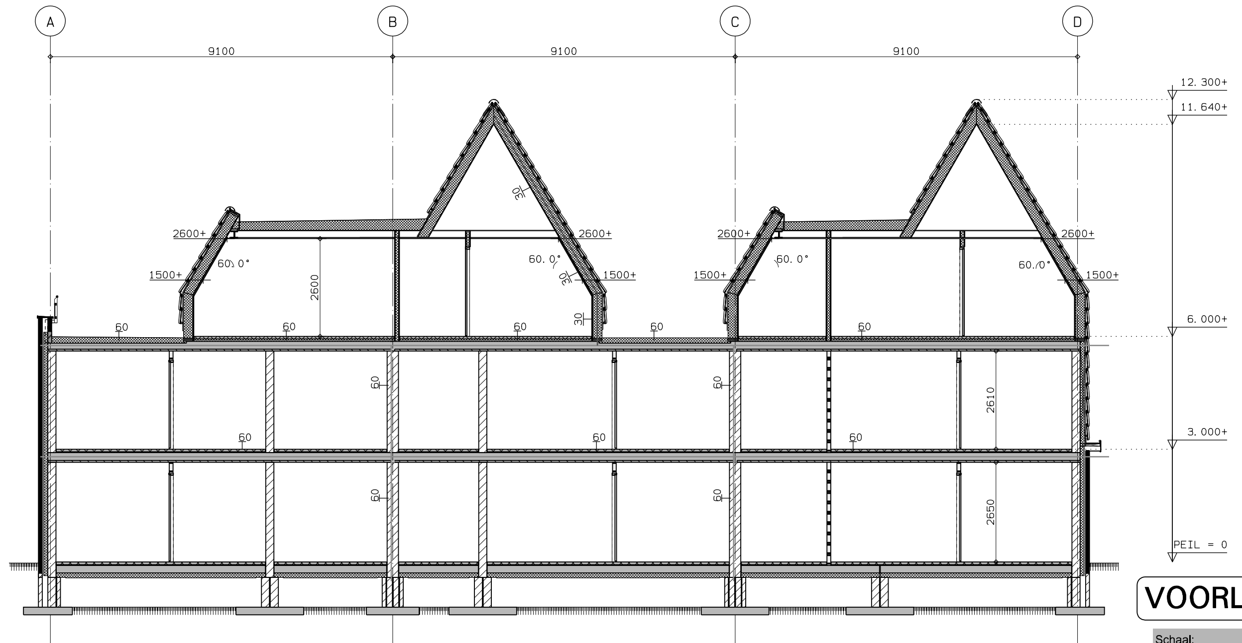
doorsnede B-B
